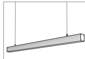
Hoogte profiel: 65 mm Breedte profiel: 49 mm Lengte: variabel
